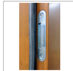
AUSHEBESICHERUNGEN 2 Stück an Bandsseite montiert Stahl, Farbe Topzink
