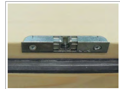
SCHNÄPPER Halter optional mit ETÖ, AV3, EAV3 Verr. Oben montiert!
