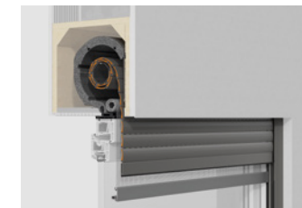
Sanierungsrollladen TERMO.F
